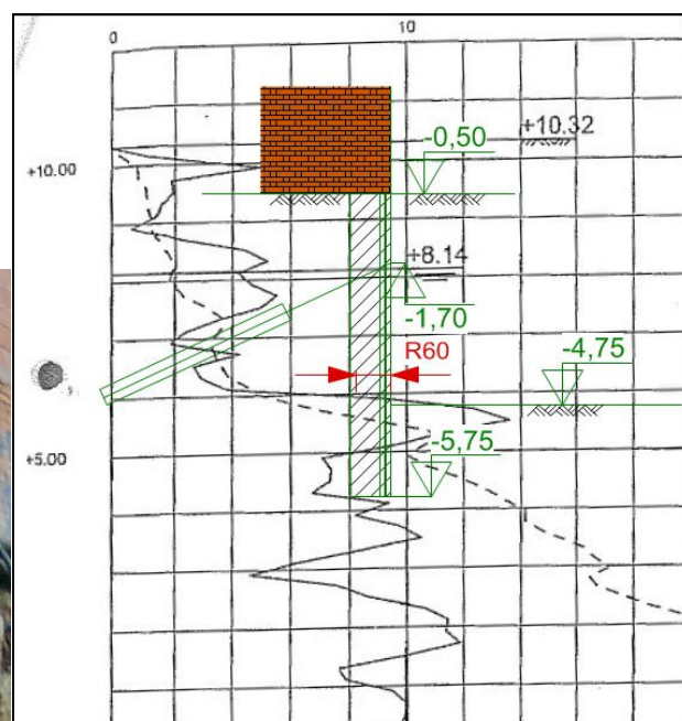
Verankerde VHP-onderschoeiing als beschoeiing van de bouwput.
