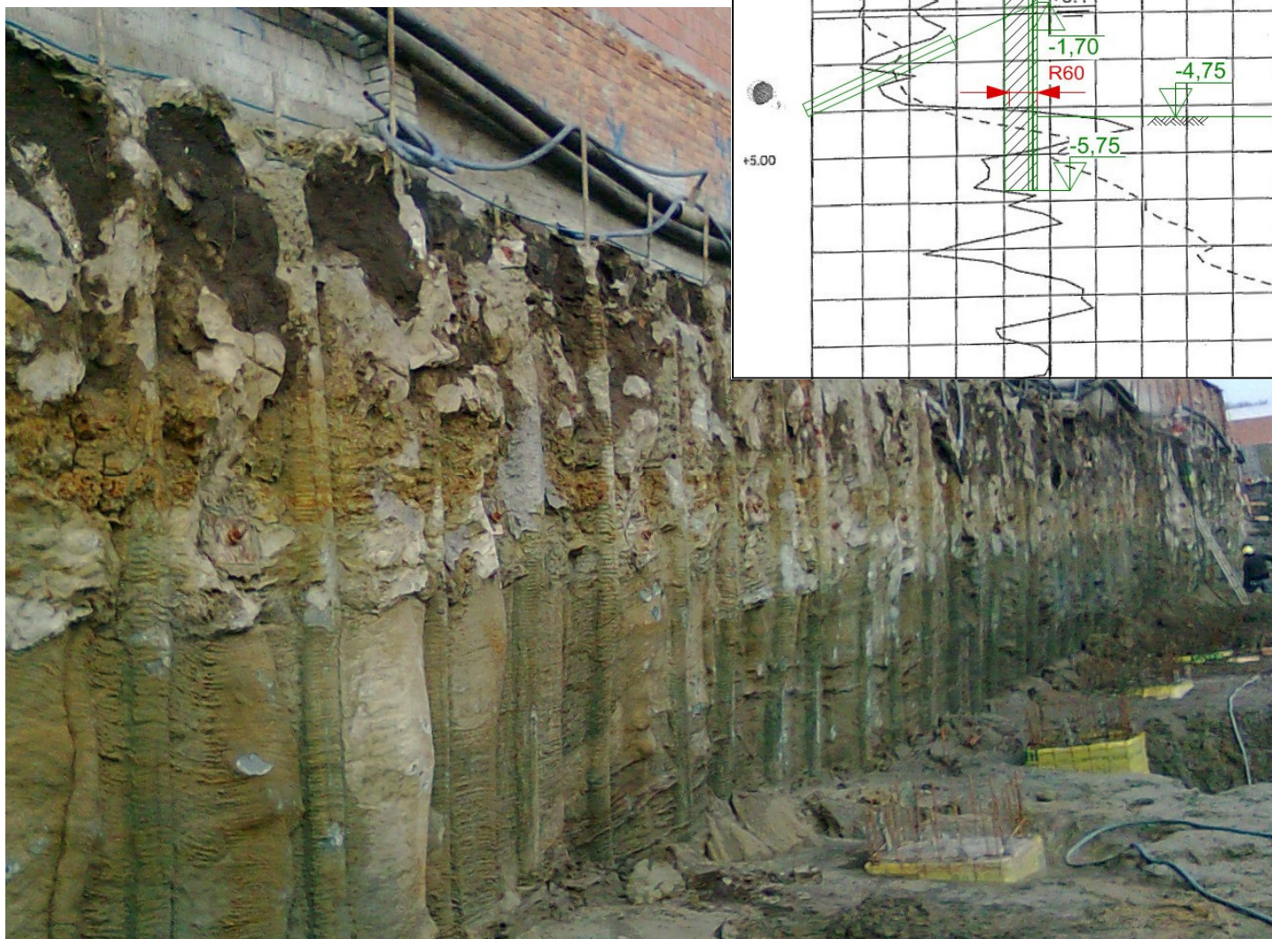
Verankerde VHP-onderschoeiing als beschoeiing van de bouwput.
